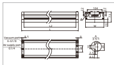
TXC130×400/600/800-A Sponge type
