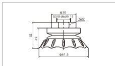
STP60□-G3F
