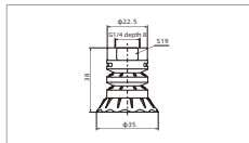
STP35□-G2F
