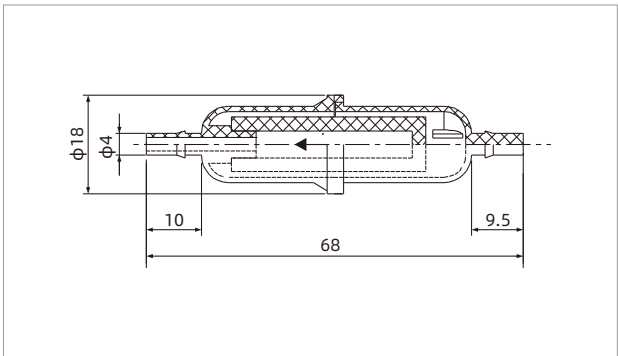
ZFL06
