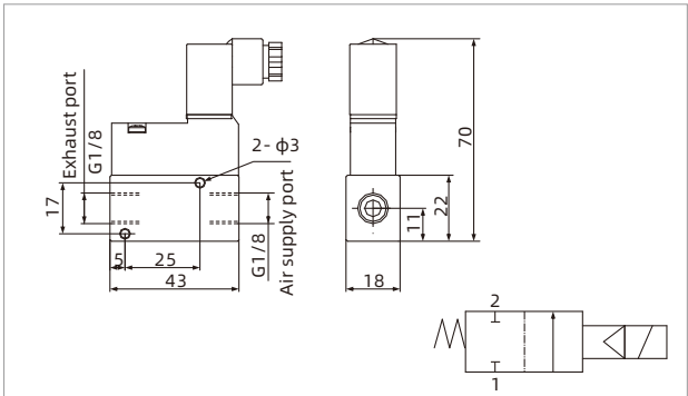
ZVEA-G1F
