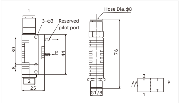
ZVAC-NO
