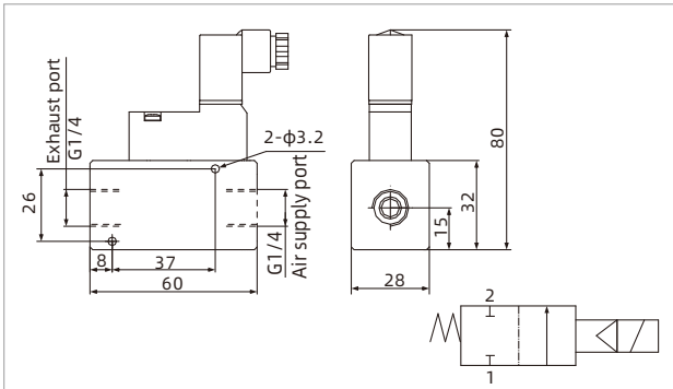
ZVEA-G2F
