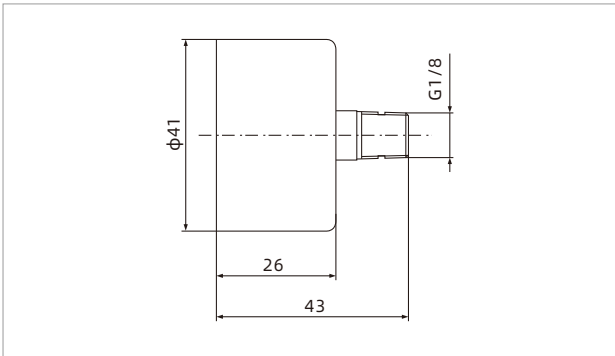
ZPMR-V
