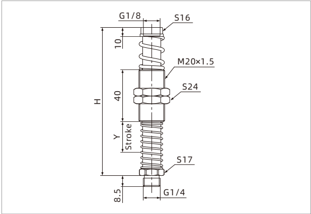
PSPD-E□(R)G2M-M20
