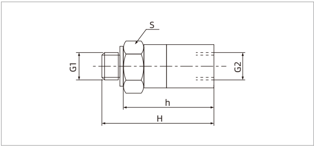
ZVRM
