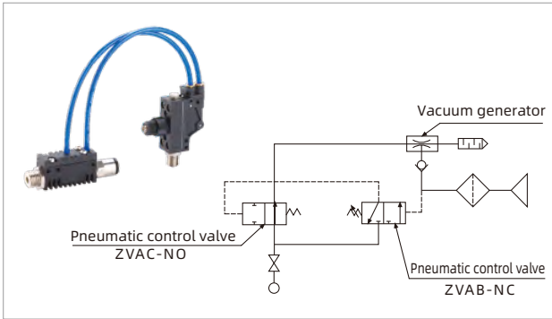
ZVU-ES
