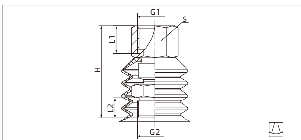
PJB-□-S
