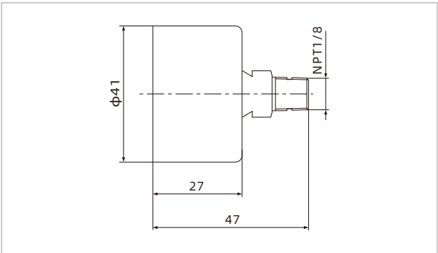
ZPMR-P
