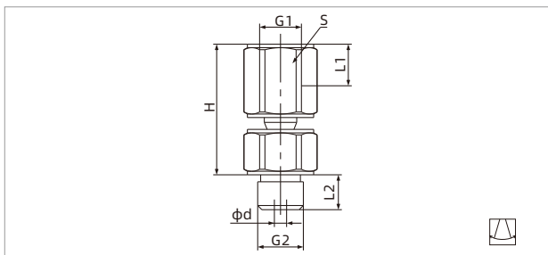
PJB-□
