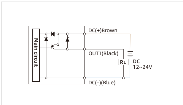
ZPDE-□P-R1M 1PNP output
