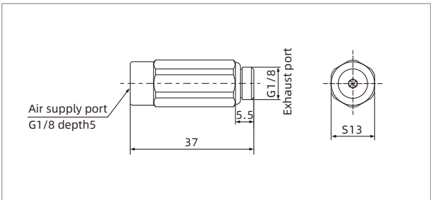
ZVS-G1F
