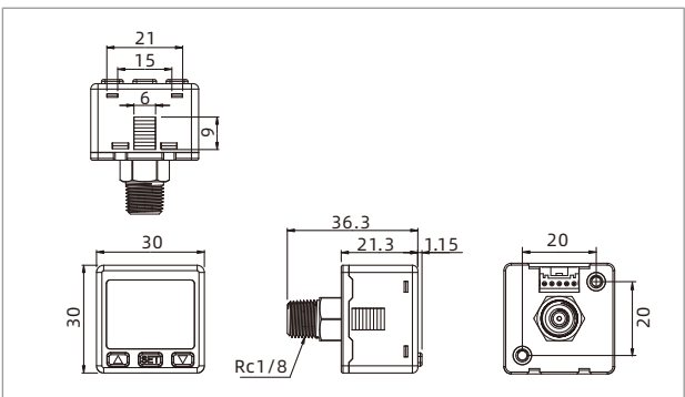
ZPDE-□N-R1M
