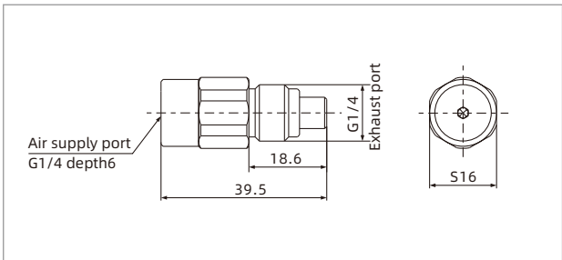
ZVS-G2F
