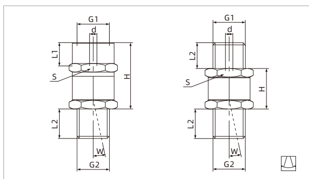
PJE-F-M
