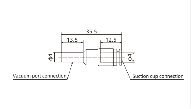
ZFD04
