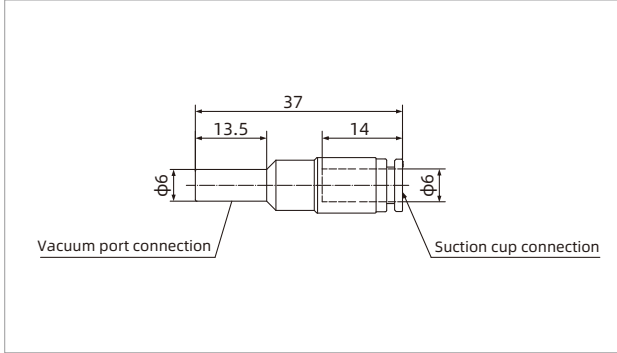
ZFD06
