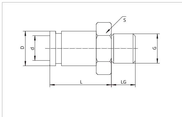
PJP-I-A8-□
