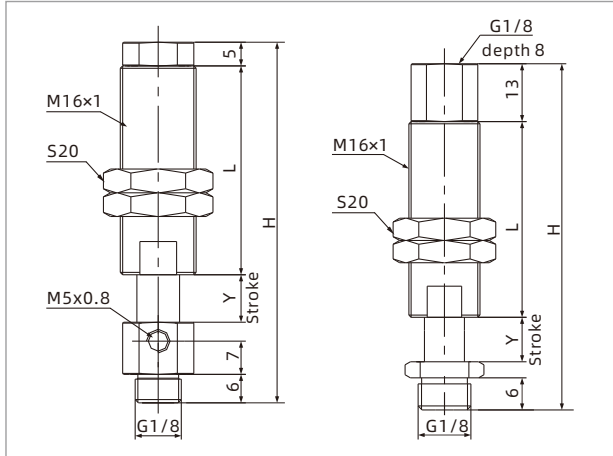
PSPT-I□LM5G1M-M16
