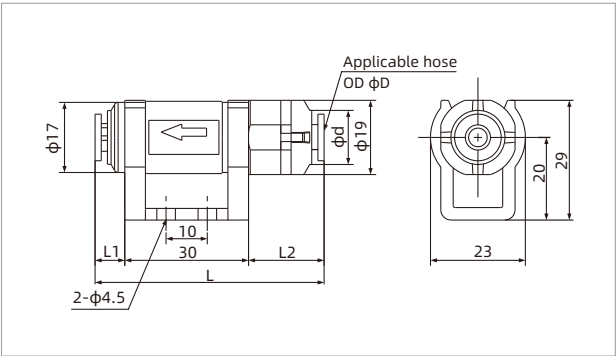
ZFA5□B
