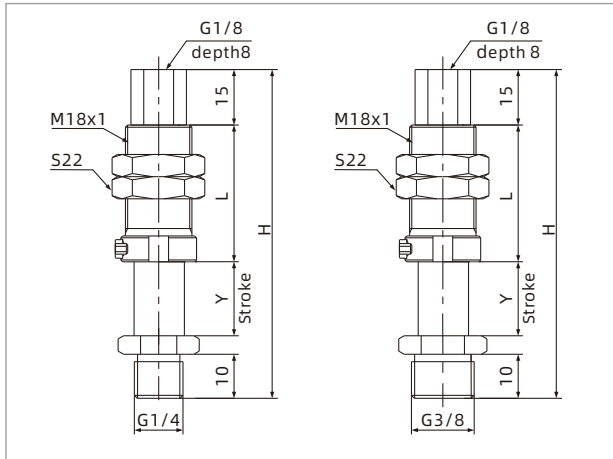
PSPT-I□RG2M-M18
