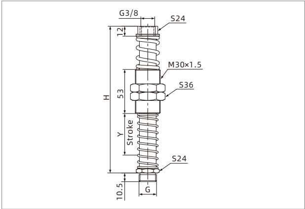
PSPD-E□(R)G3M-M30 PSPD-E□(R)G4M-M30
