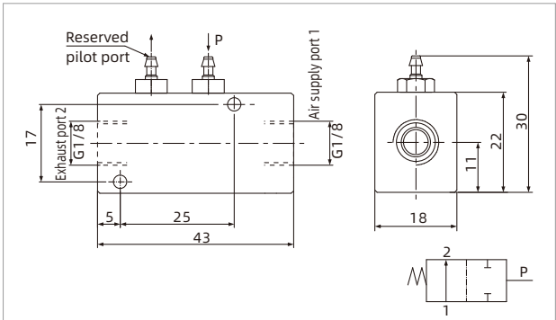
ZVAA-G1F
